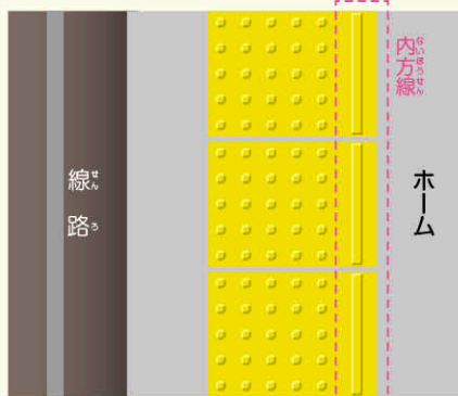
内方線付き点字ブロック
